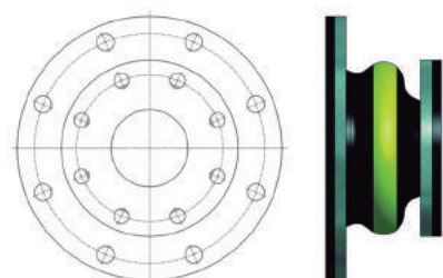
Concéntricos (ejes alineados)
